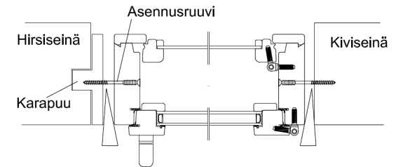
Kuva 2. Avattavan ikkunan asennus karpuuhun tai kiviseinään.
