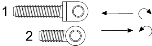
Kuva 1. Haarukka-(1) ja holkkiosan (2) säätäminen.
